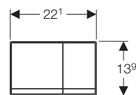
Geberit Sigma60, placca di comando Art. 115.792.GH.1
